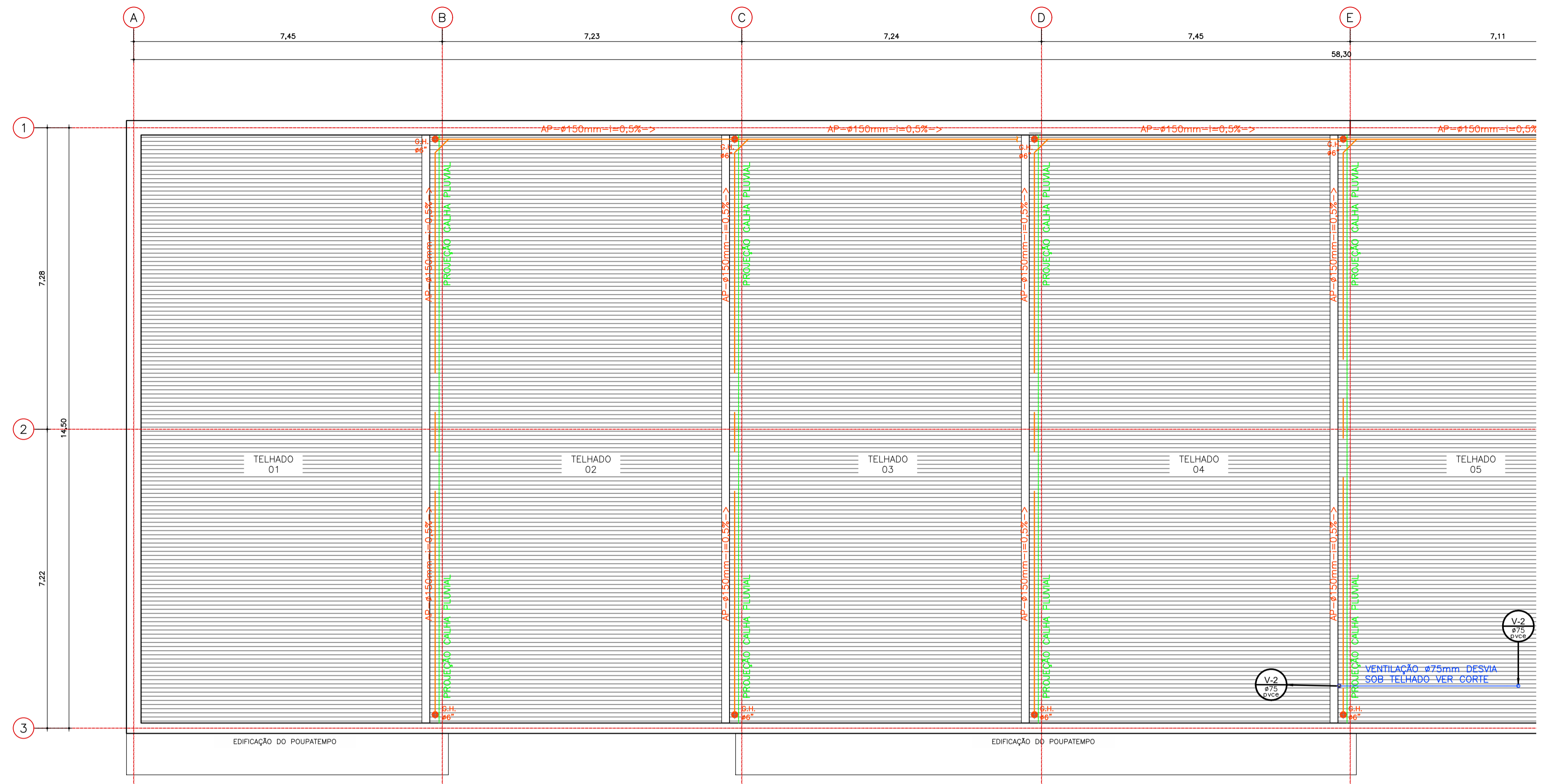
EDIFÍCIO DEFENSORIA PÚBLICA COBERTURA REDES PLUVIAIS E DESVIOS DE VENTILAÇÕES ESCALA 1:75
