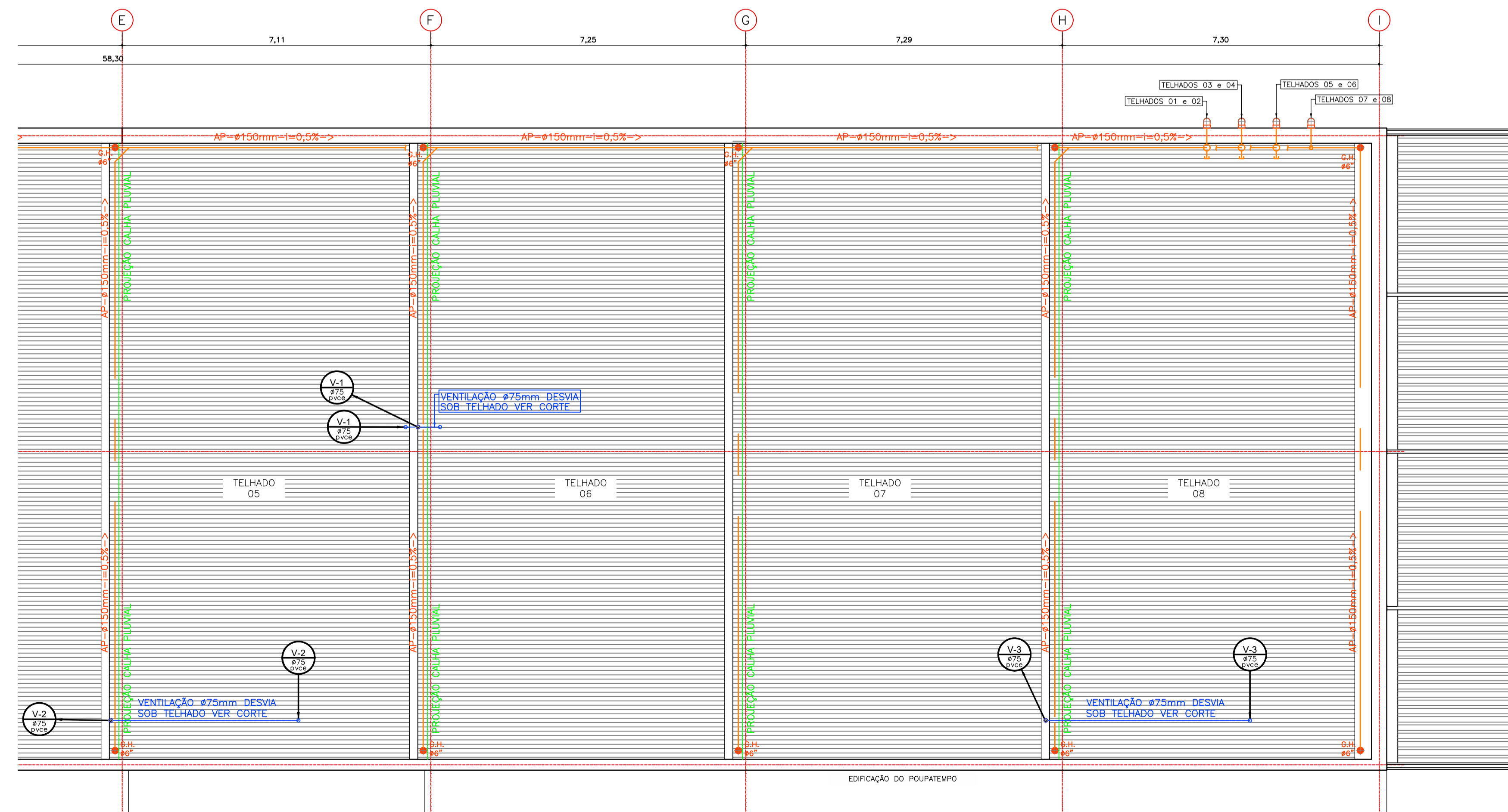
EDIFÍCIO DEFENSORIA PÚBLICA COBERTURA REDES PLUVIAIS E DESVIOS DE VENTILAÇÕES ESCALA 1:75
