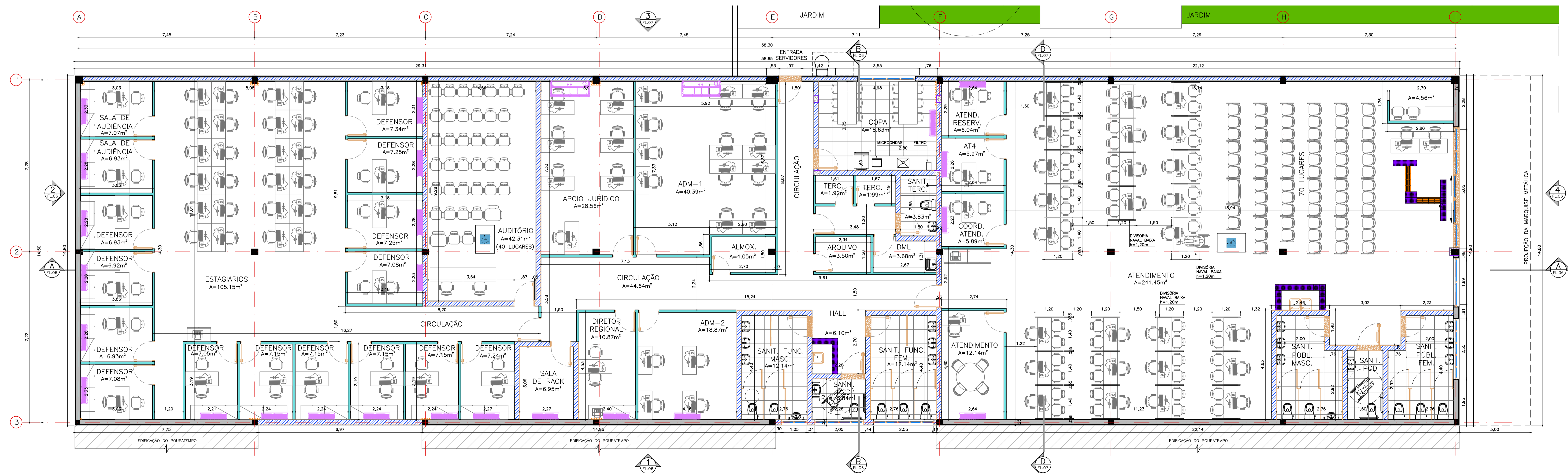
EDIFÍCIO DEFENSORIA PÚBLICA PLANTA PAV. TÉRREO – LAYOUT ESCALA 1:75
