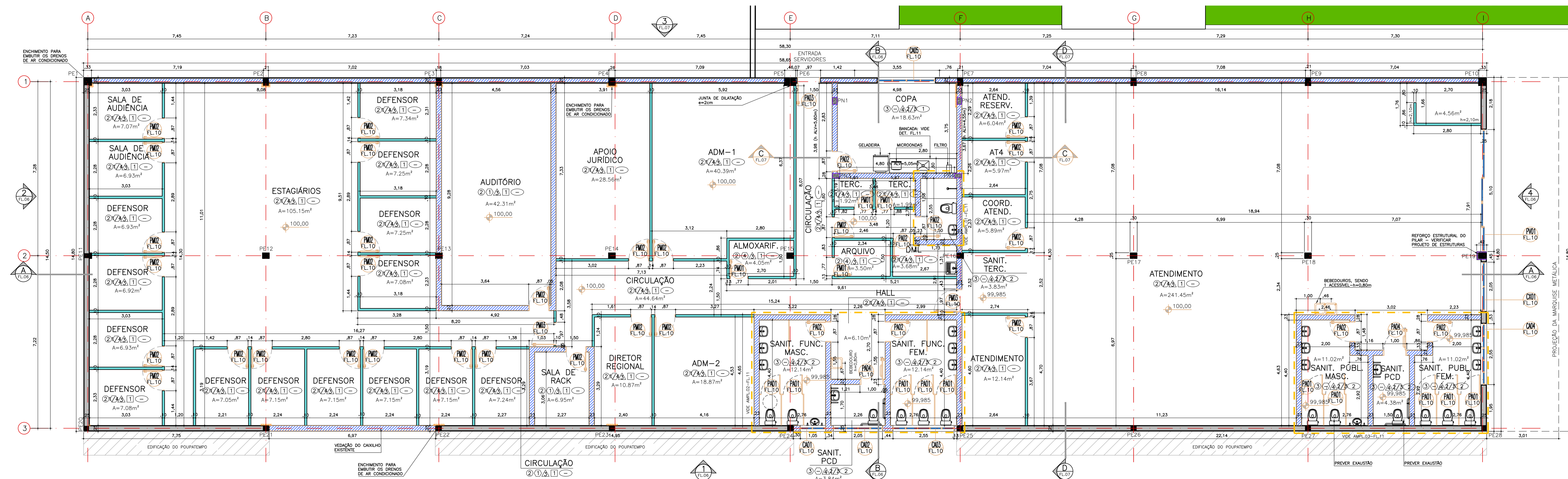
EDIFÍCIO DEFENSORIA PÚBLICA PLANTA PAV. TÉRREO - CONSTRUÇÕES ESCALA 1:75
